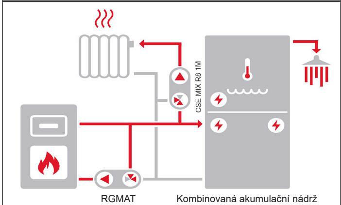
Příklad zapojení II
