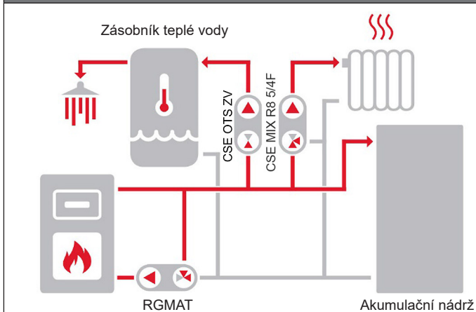
Příklad zapojení I
